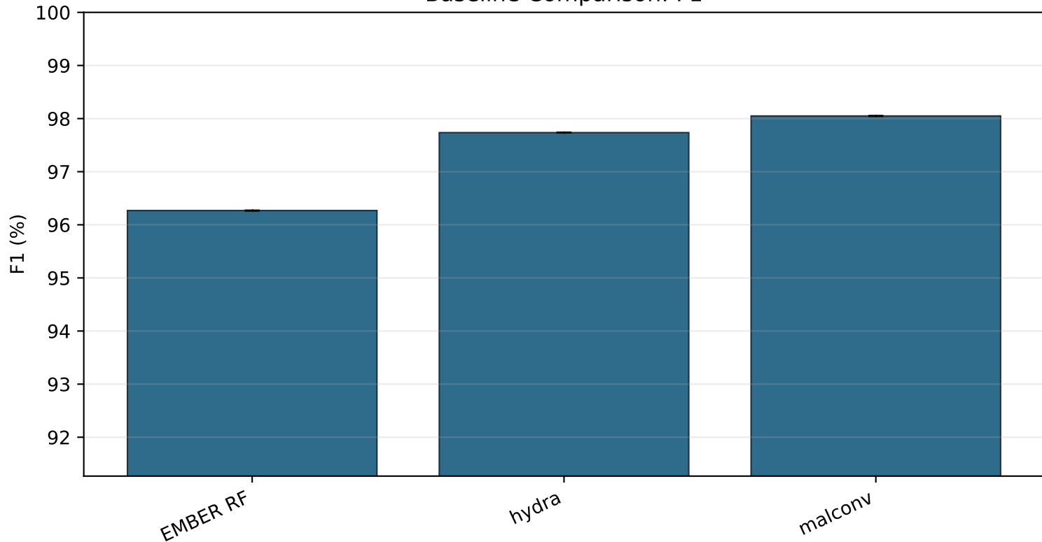
Baseline Comparison: F1
