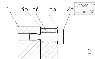
Detail 1, Schnitt (1:1)
