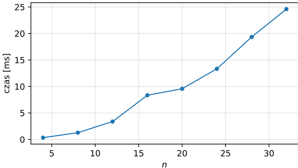
qr_givens: czas jednego wywołania
