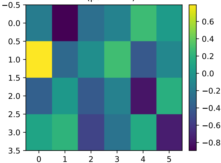
V^T (path AA^T )
