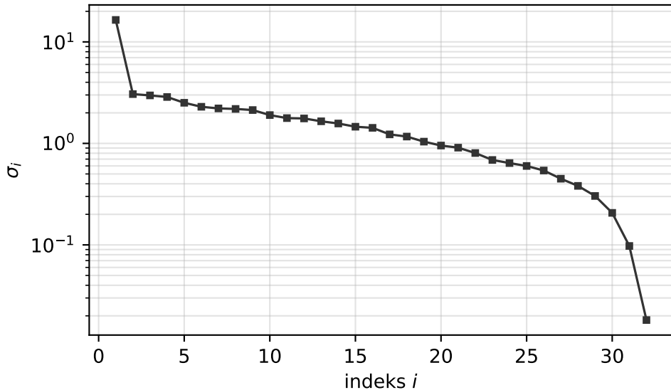
Wartosci osobliwe macierzy M ( n \times n )
