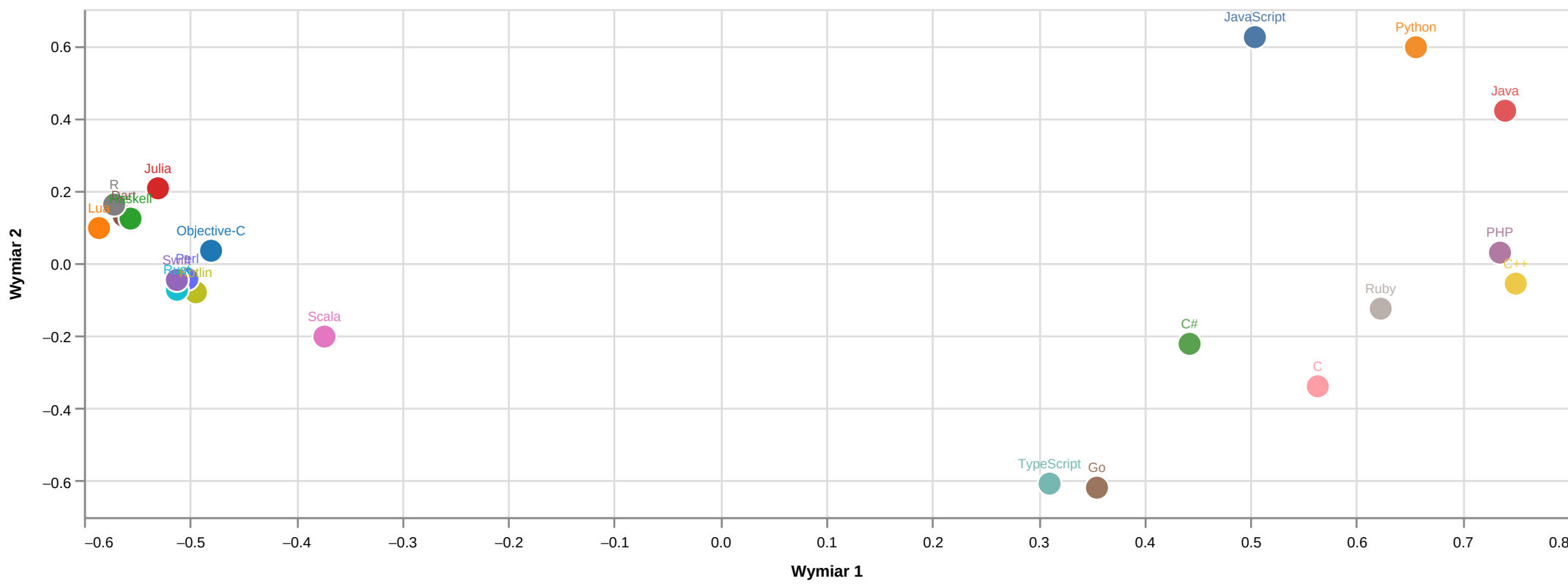
t-SNE (sklearn)
