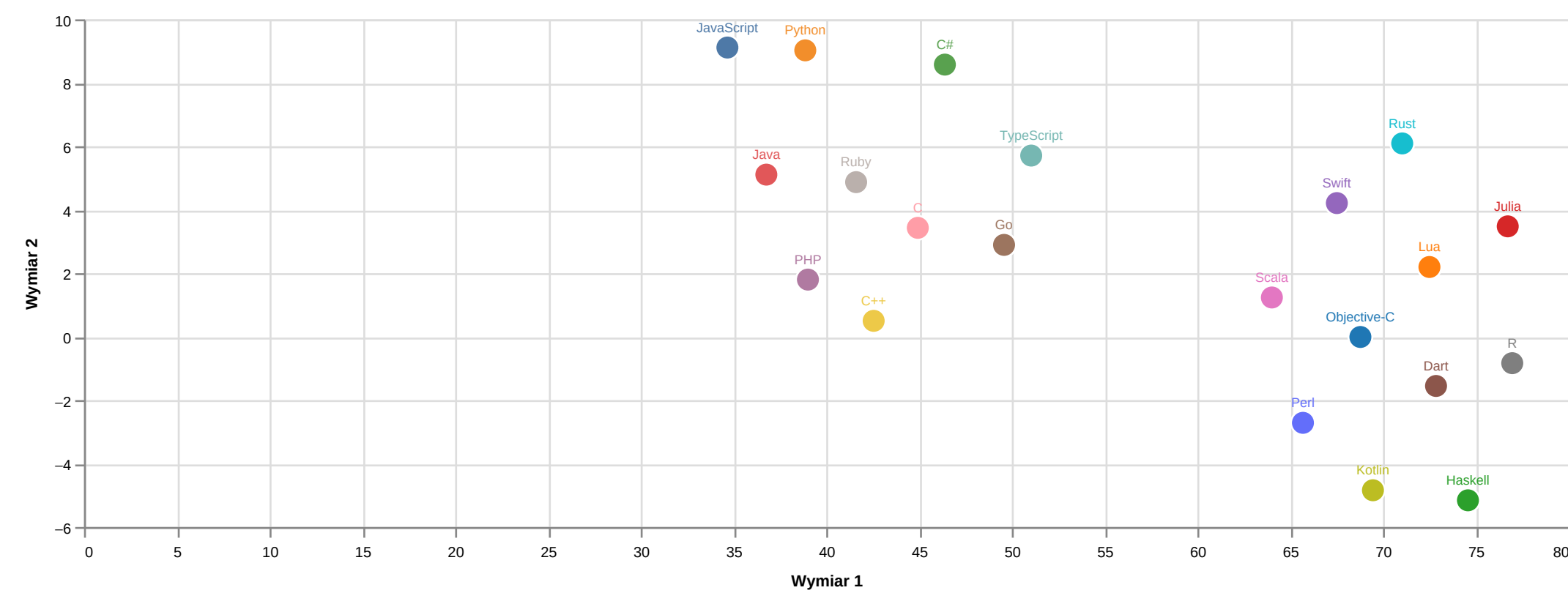
UMAP
