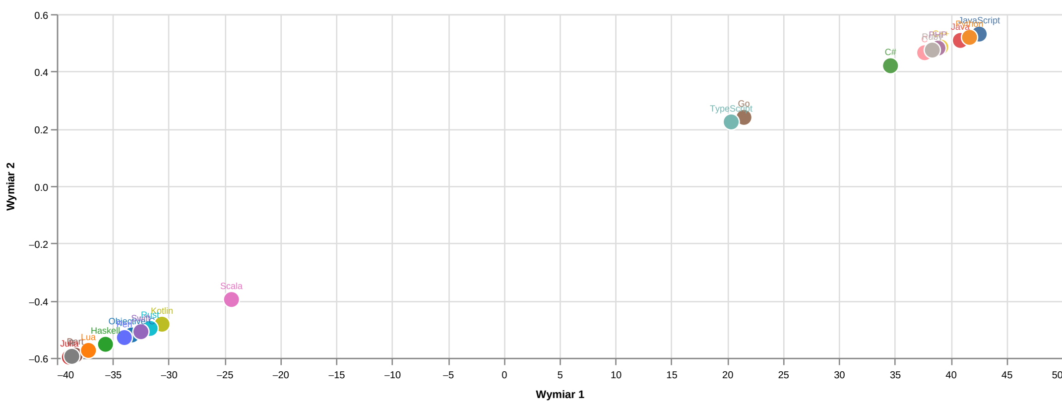
PaCMAP
