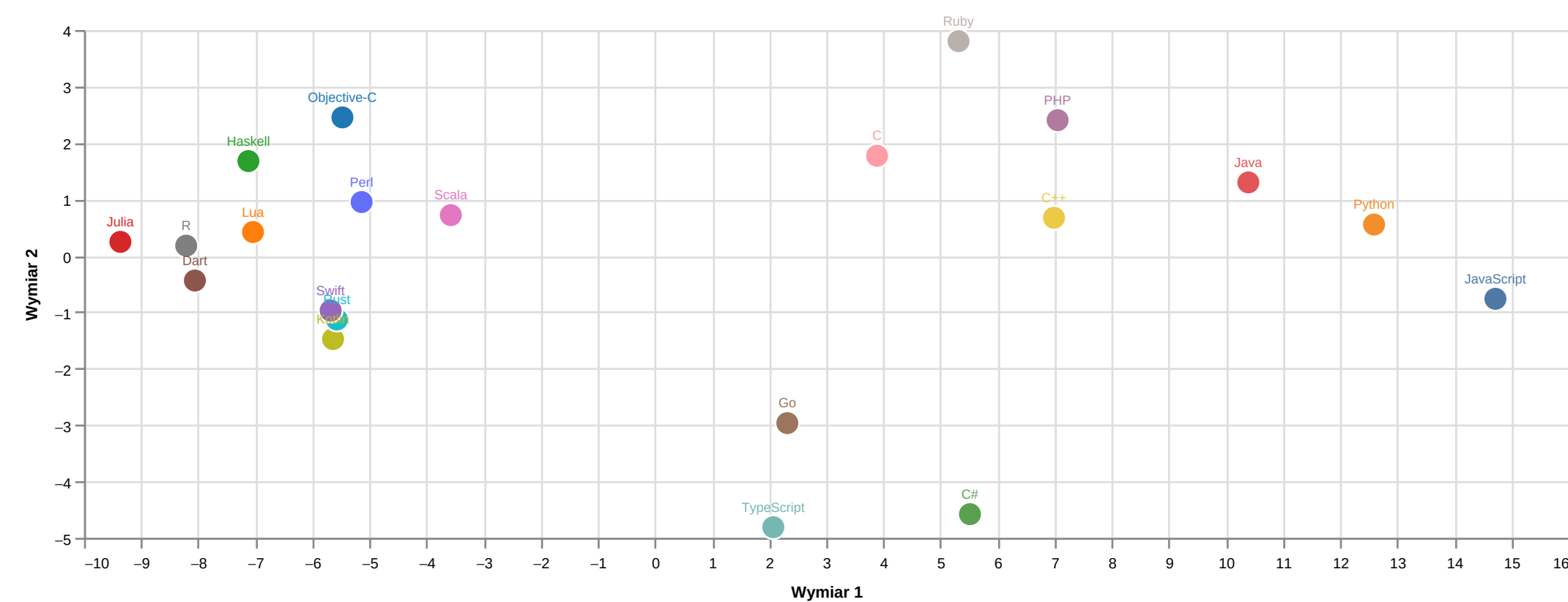
PCA
