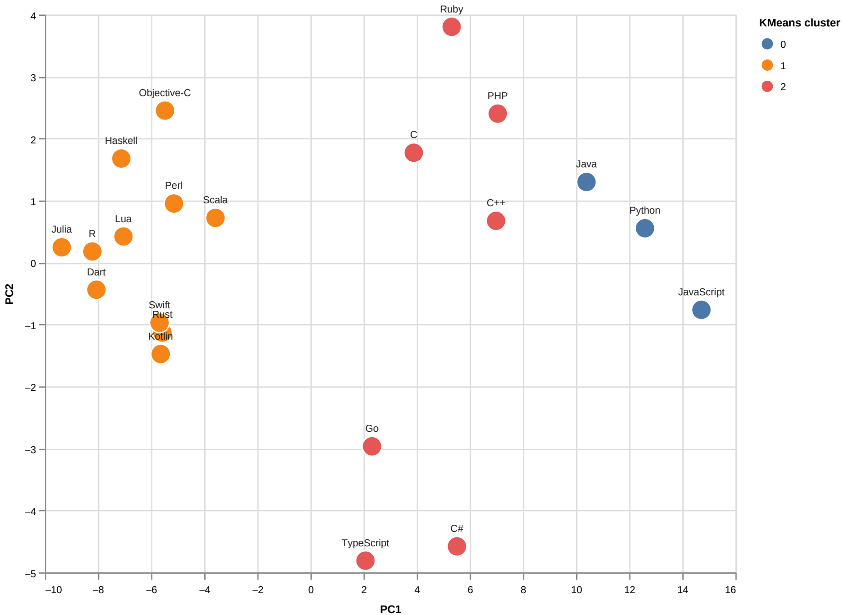
EDA: k-means clusters on PCA space (k=3)
