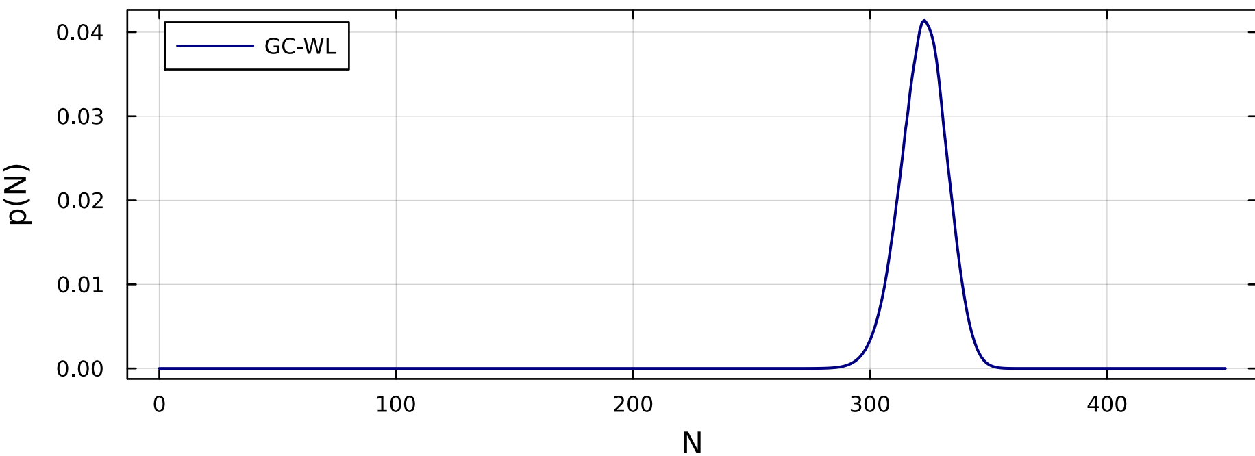
(b) \mu = -361.68 kJ/kg (bulk vapor)
