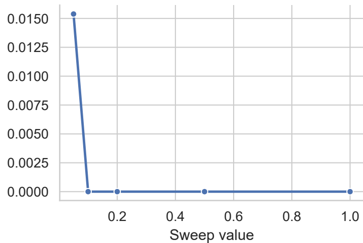
Linear TS
