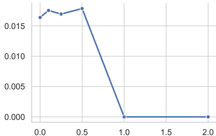
Linear TS
