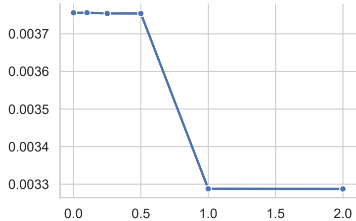
Linear TS
