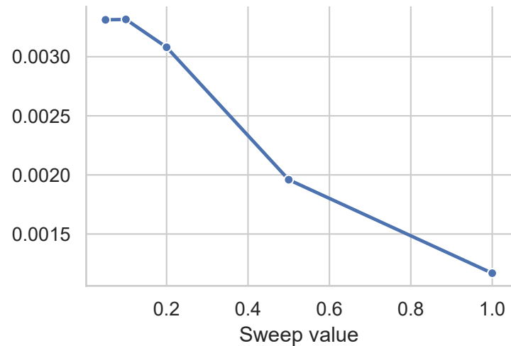
Linear TS
