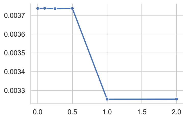
Linear TS
