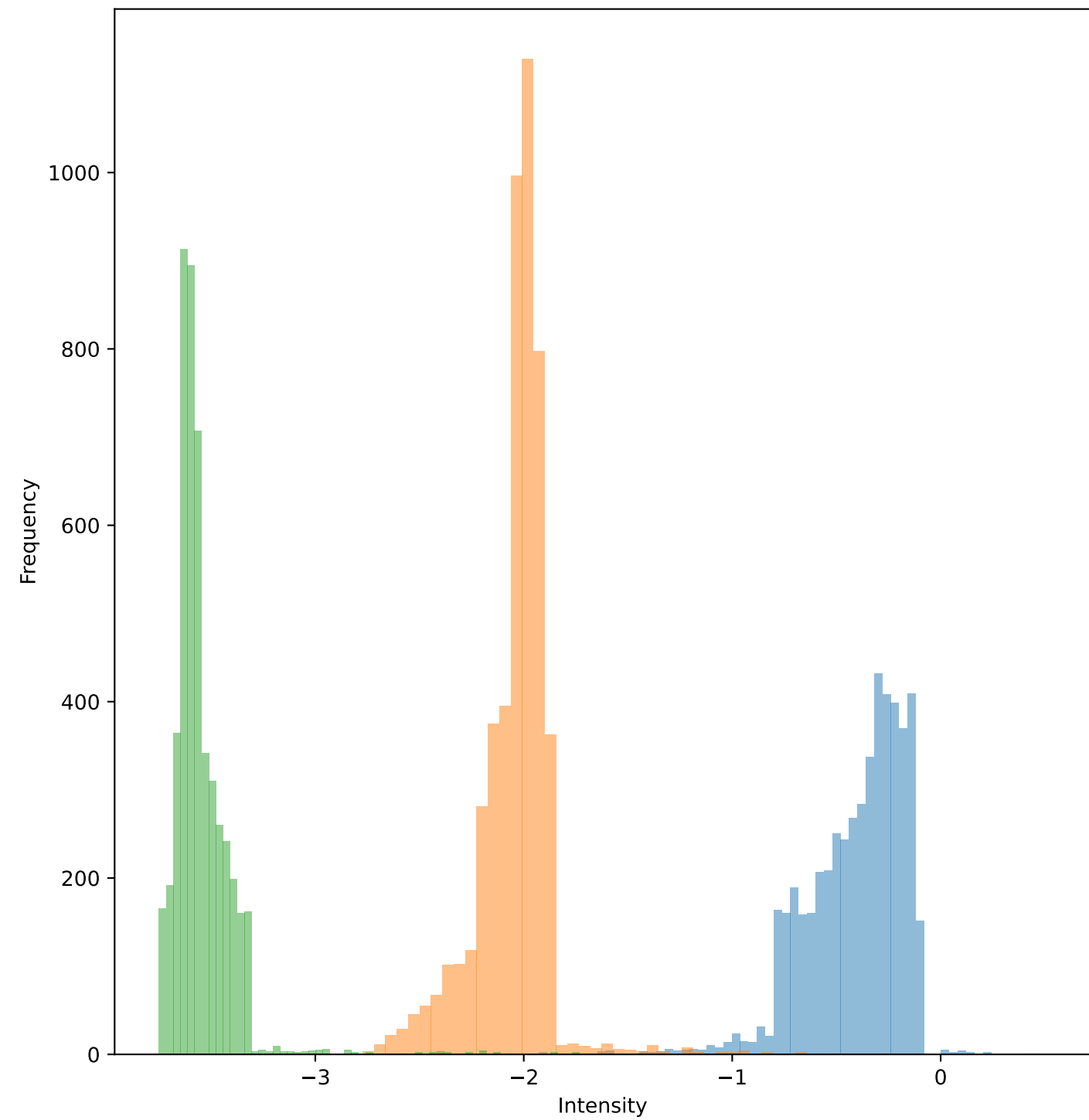
CLIN (Ours)
