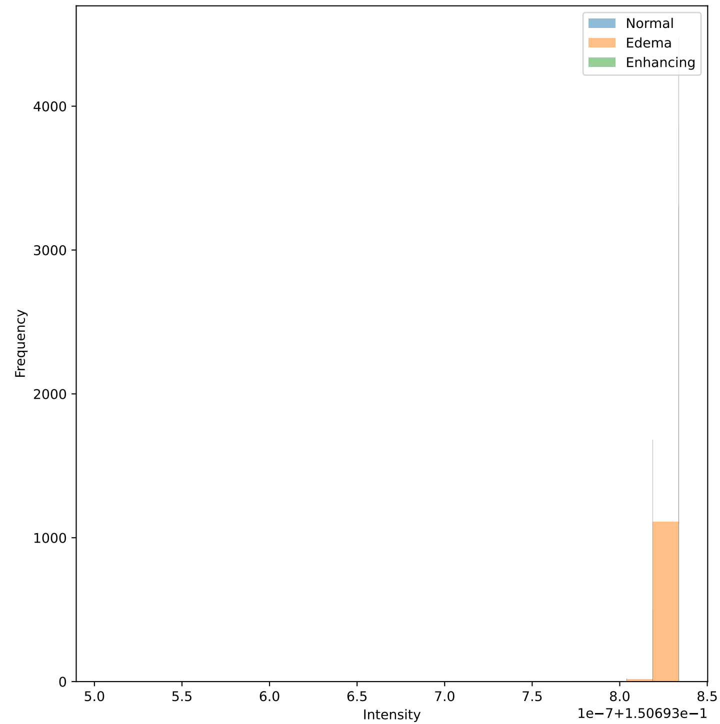
Uncond. LIN
