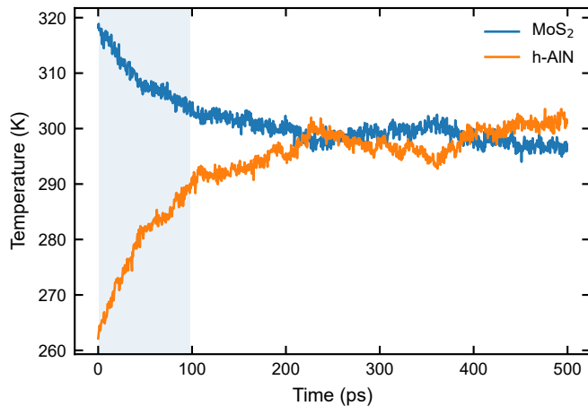
(d) Representative layer temperatures
