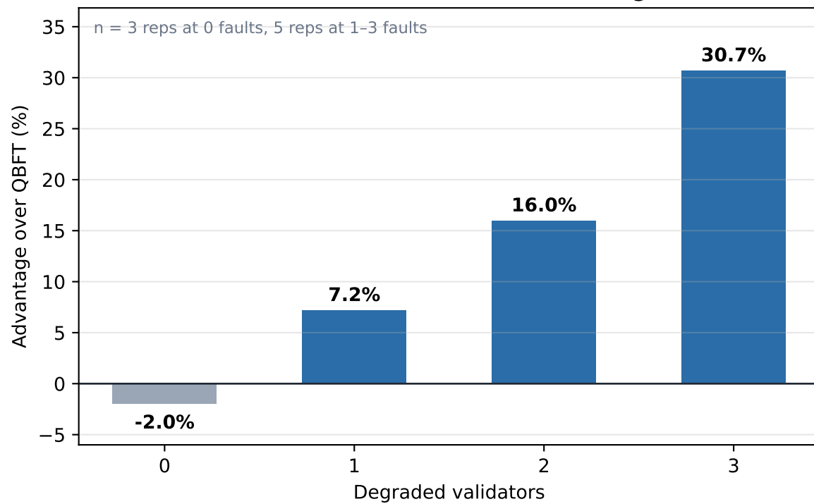
(d) CB-BFT block-interval advantage
