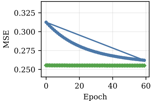
XOR — Loss
