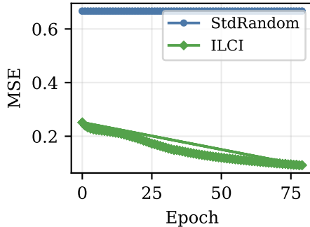
Iris — Loss
