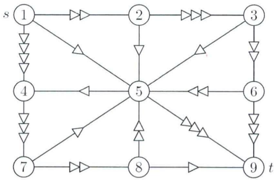
Flot au début de la 7 e itération
