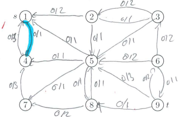
Sixième réseau d'augmentation du flot
