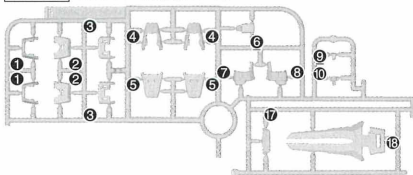
E/パーツ (スチロール樹脂: PS)
