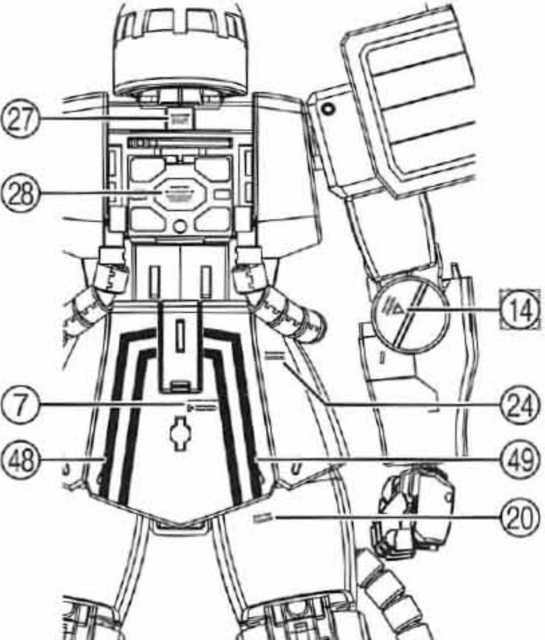
<ボディ内装背面> <Body interior back side>
