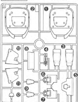
Fパーツ (スチロール樹脂: PS)
