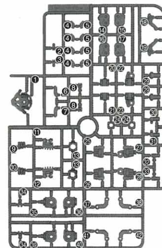
Gパーツ (グレー) (ABS樹脂: ABS)
