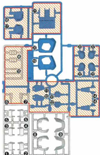
Eパーツ (ブルー・ホワイト) (スチロール樹脂: PS)
