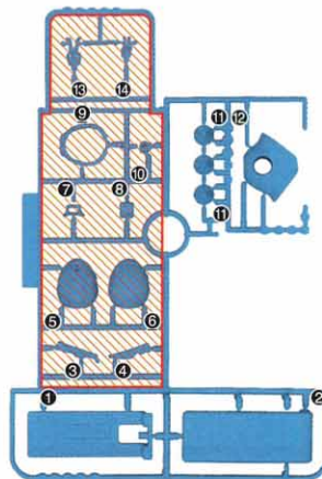
Dパーツ (ブルー) (スチロール樹脂: PS)
