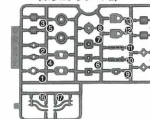
<PC-200A> (グレー) (ポリエチレン: PE)
