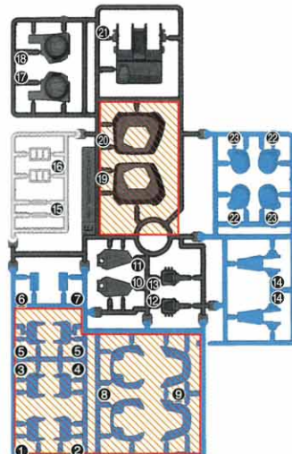
Eパーツ (ダークグレー・ブルー・ホワイト) (スチロール樹脂: PS)
