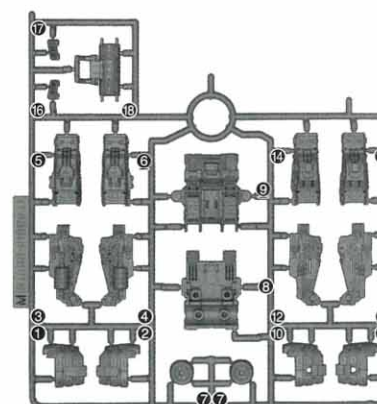
Mパーツ (グレー) (スチロール樹脂: PS)
