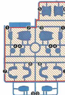
Fパーツ (グレー) (ABS樹脂: ABS)
