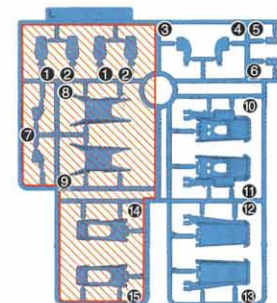
Lパーツ (ブルー) (スチロール樹脂: PS)
