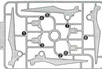
デスティニー Gパーツ(パープル) (スチロール樹脂: PS)
