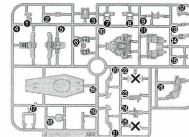
Jパーツ(グレー) (ABS樹脂: ABS) アンダーゲート有D
