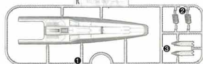
Kパーツ(ホワイト) (スチロール樹脂: PS)
