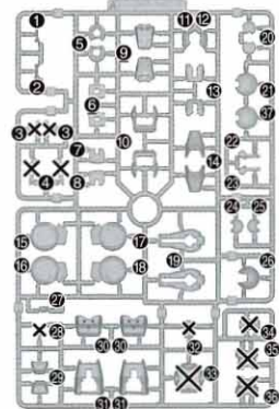
Eパーツ(グレー) (スチロール樹脂: PS)
