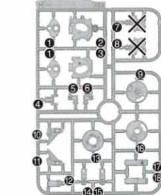
Hパーツ(グレー) アンダーゲート有り (ABS樹脂: ABS)
