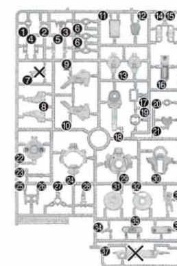
U1パーツ(クリアグリーン) (スチロール樹脂: PS)
