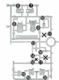
N2パーツ(イロプラ) (スチロール樹脂: PS)
