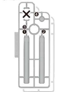
Iパーツ(ライトグレー) I Parts (Light gray) (PS) (×2)
