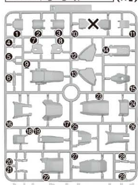
Dパーツ(ライトグレー) (PS) D Parts (Light gray) (×2)
