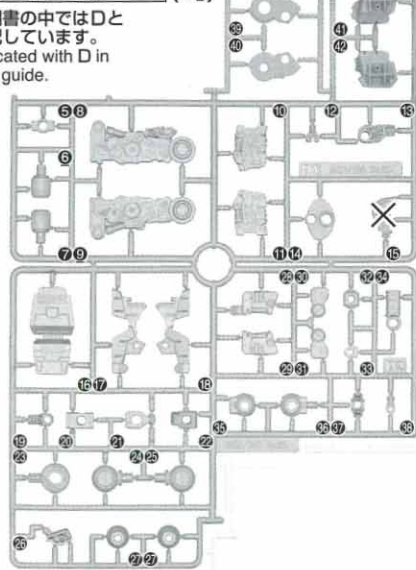
D1・D2パーツ(グレー) (PS) D1・D2 Parts (Gray) (x 2)
