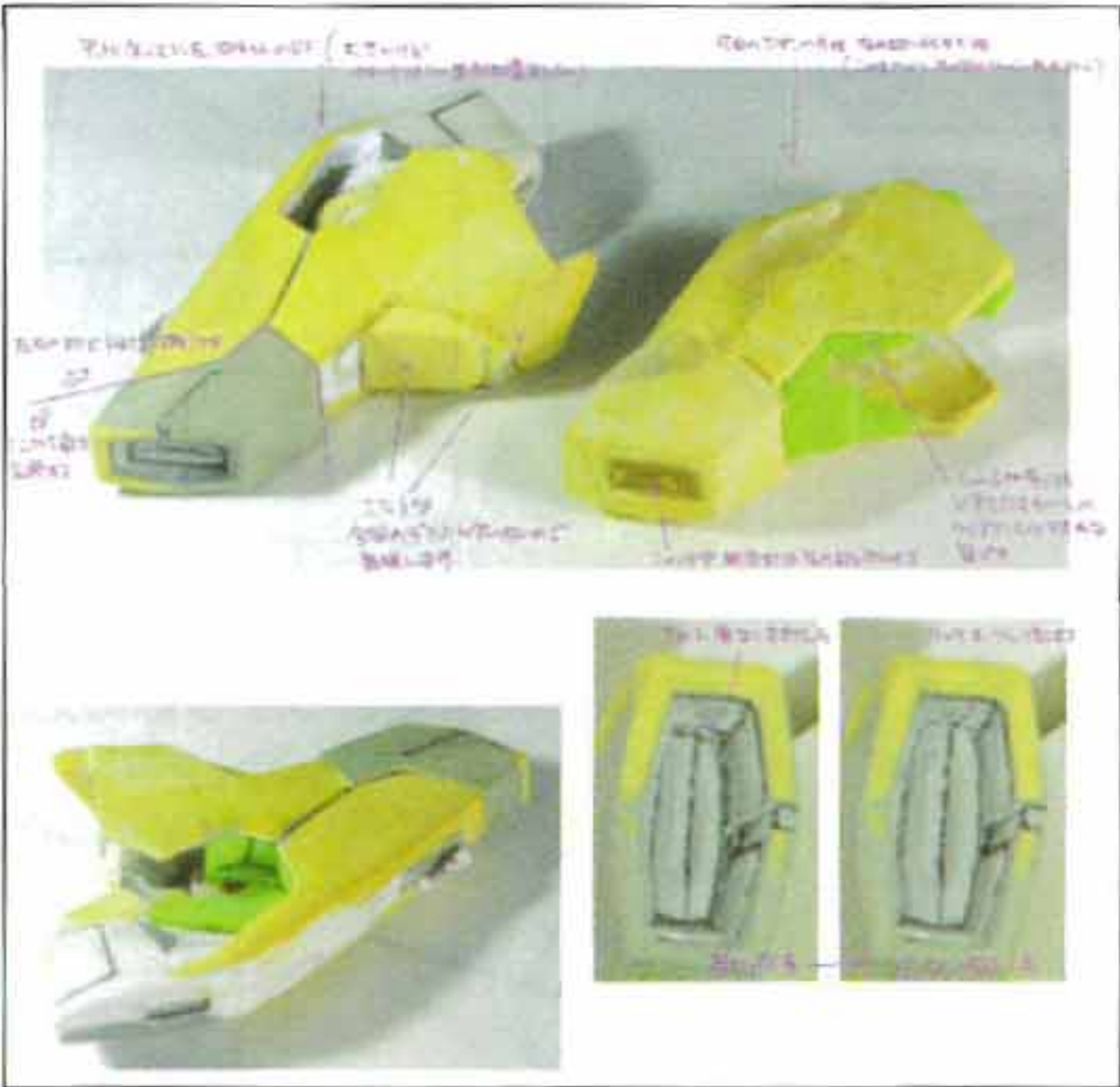
写真上は左が旧キットをベースに先に作ったもの、右が今回の試作品をベースに形状を修正したもの。旧キットベースは六角形になっており、それを今回のMG Ver.Kaでも取り入れている
