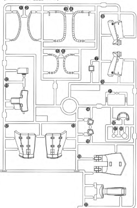
Aパーツ (スチロール樹脂：PS)
