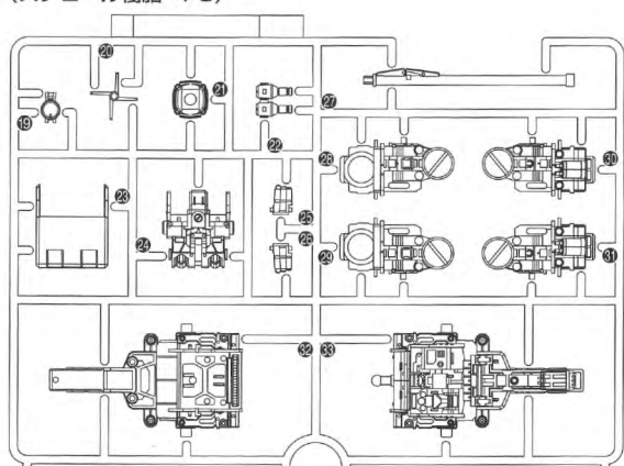
B2パーツ (スチロール樹脂：PS)
