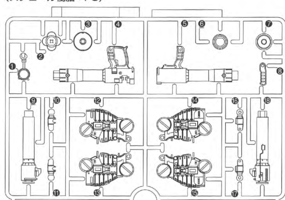
B1パーツ (スチロール樹脂：PS)
