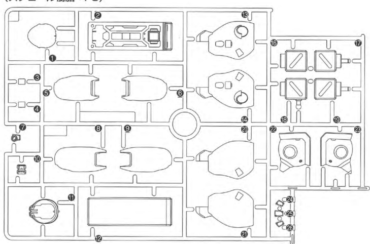
Cパーツ (スチロール樹脂：PS)
