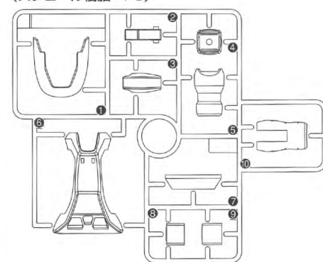
Gパーツ (×2) (スチロール樹脂：PS)
