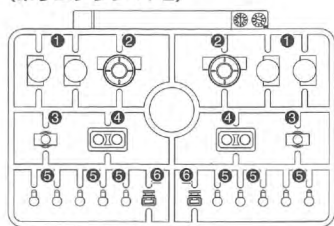
Kパーツ (ポリエチレン: PE)
