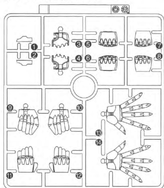
L1パーツ (スチロール樹脂: PS)
