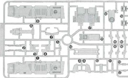
GLパーツ (ABS樹脂: ABS)
