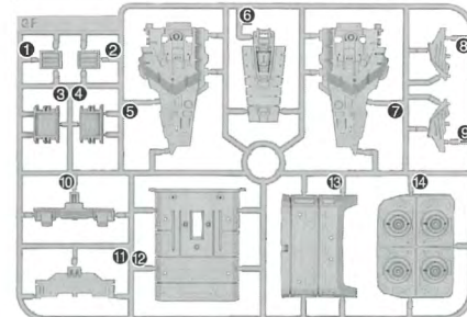
GFパーツ (スチロール樹脂: PS)
