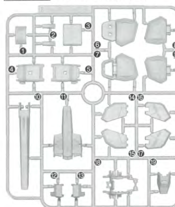
Iパーツ (スチロール樹脂: PS)
