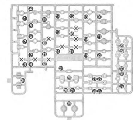
PC-207BDE(グレー) (ポリエチレン: PE)
