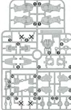
Eパーツ(グレー) (ABS樹脂: ABS)
