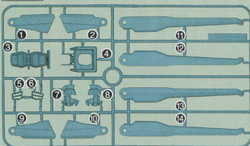
Lパーツ (スチロール樹脂: PS)
