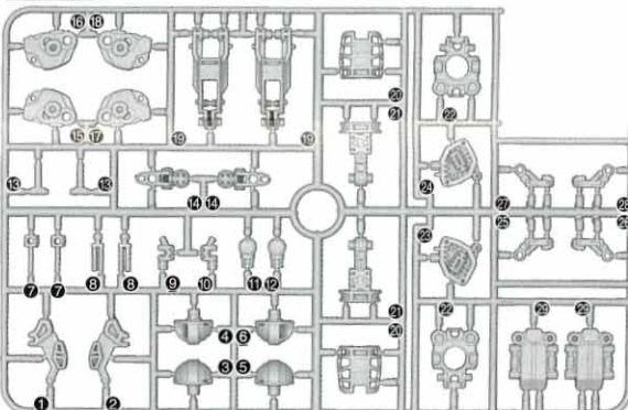
Kパーツ (スチロール樹脂: PS) (ポリエチレン: PE)
