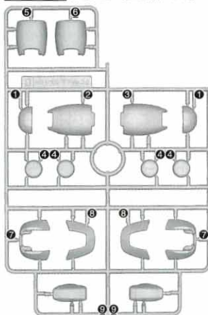
Dパーツ (スチロール樹脂: PS)
