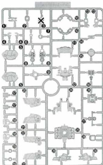
Hパーツ(グレー) (ABS樹脂: ABS)
