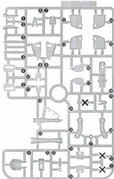
Eパーツ(ホワイト) (スチロール樹脂: PS)
