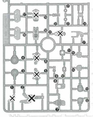
Fパーツ(グレー) (×2) (スチロール樹脂: PS)
