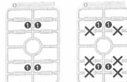
Oパーツ (×2) (スチロール樹脂: PS)
