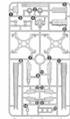
WBパーツ (×2) (スチロール樹脂: PS)
