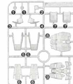
Yパーツ (ABS樹脂: ABS)
