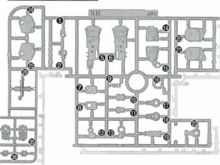
XBパーツ(グレー) (X2) (ABS樹脂: ABS)
