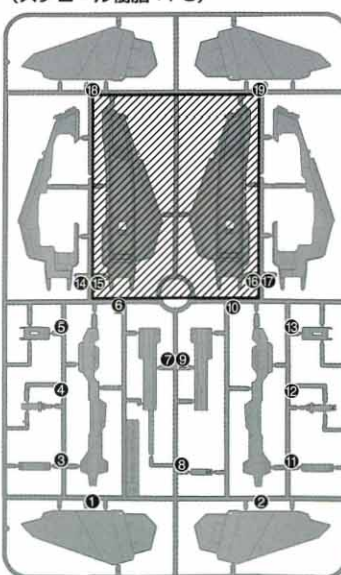
Gパーツ(オレンジ) (スチロール樹脂: PS)
