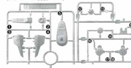
アンダーゲート有り (スチロール樹脂: PS)
