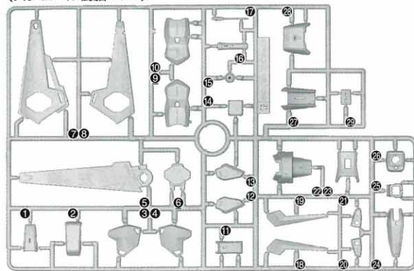
アンダーゲート有り (スチロール樹脂: PS)
