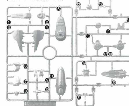
アンダーゲート有り (スチロール樹脂: PS)
