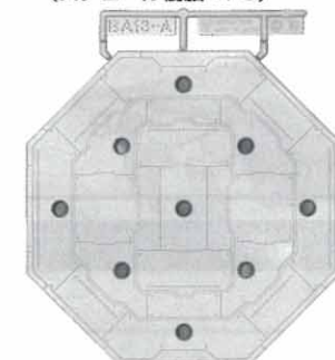
BA13-Aパーツ(ブラック) (スチロール樹脂: PS)
