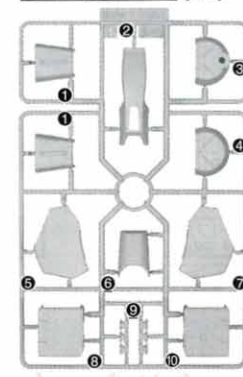
Iパーツ(ブルー) (PS) I Parts (Blue) (×2)
