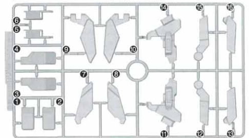
WUパーツ(ホワイト) (PS) WU Parts (White)
