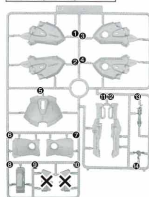
F1パーツ(ダークレッド) (PS) F1 Parts (Dark red)
