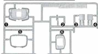
A1パーツ(ライトグリーン) (PS) A1 Parts (Light green)
