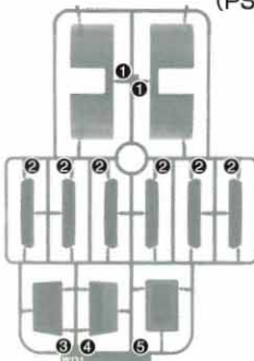
WD1パーツ(ライトグレー) WD1 Parts (LIGHT GRAY) (PS)
