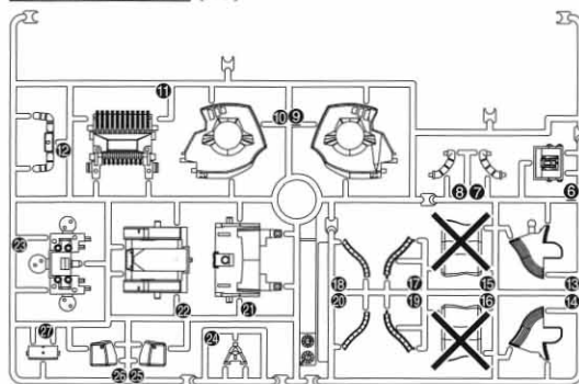
Cパーツ(ホワイト) (PS) C Parts (White) (×2)
