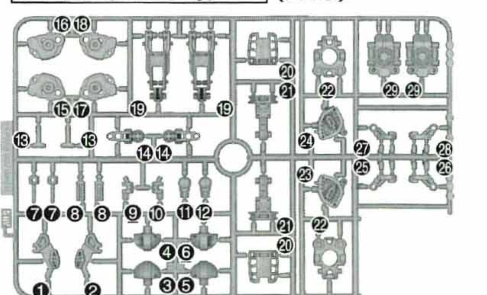
Hパーツ(ダークグレー) H Parts (Dark Gray) (ABS)
