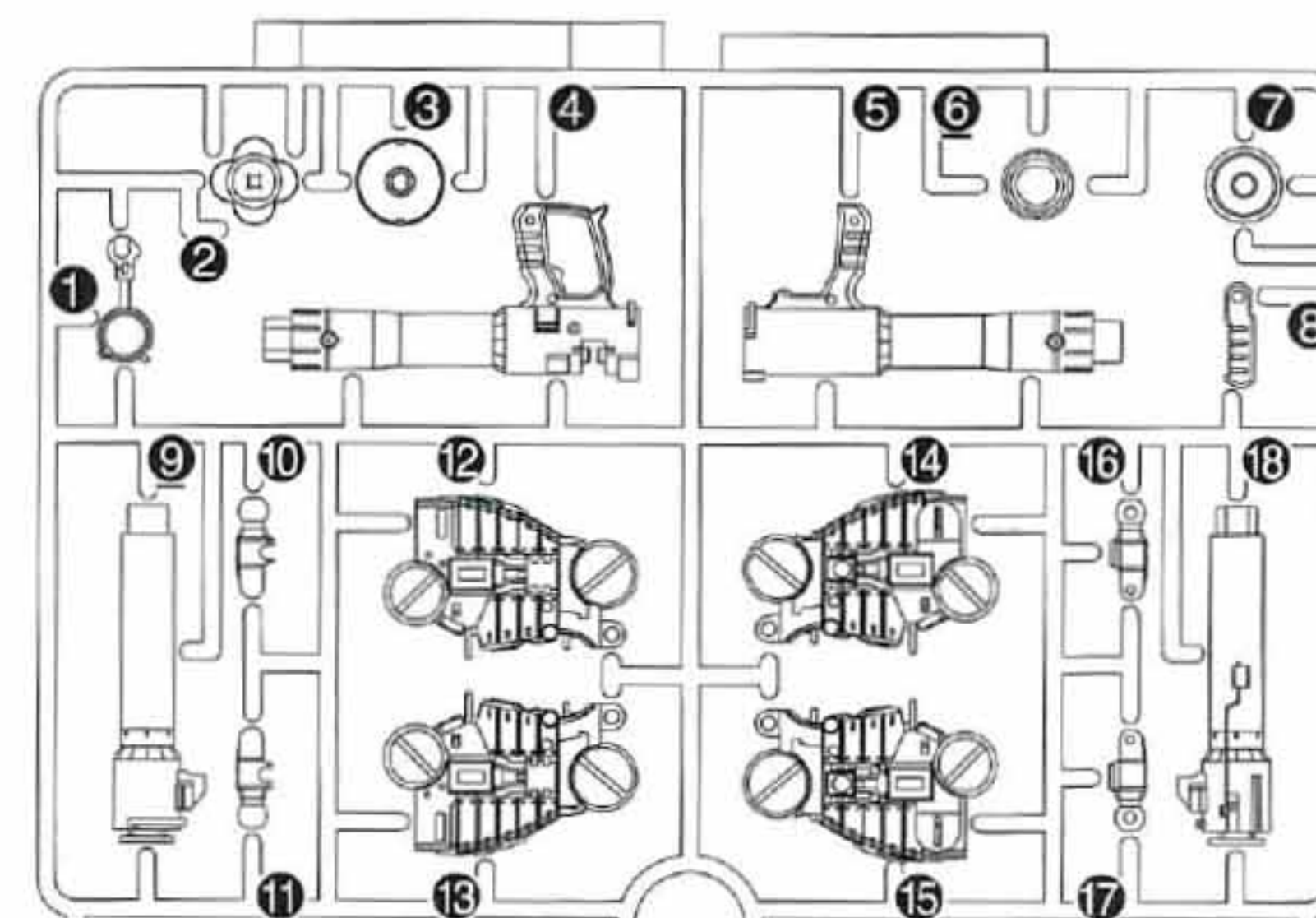
B1パーツ(ブルーグレー) (PS) B1 Parts (Blue Gray)
