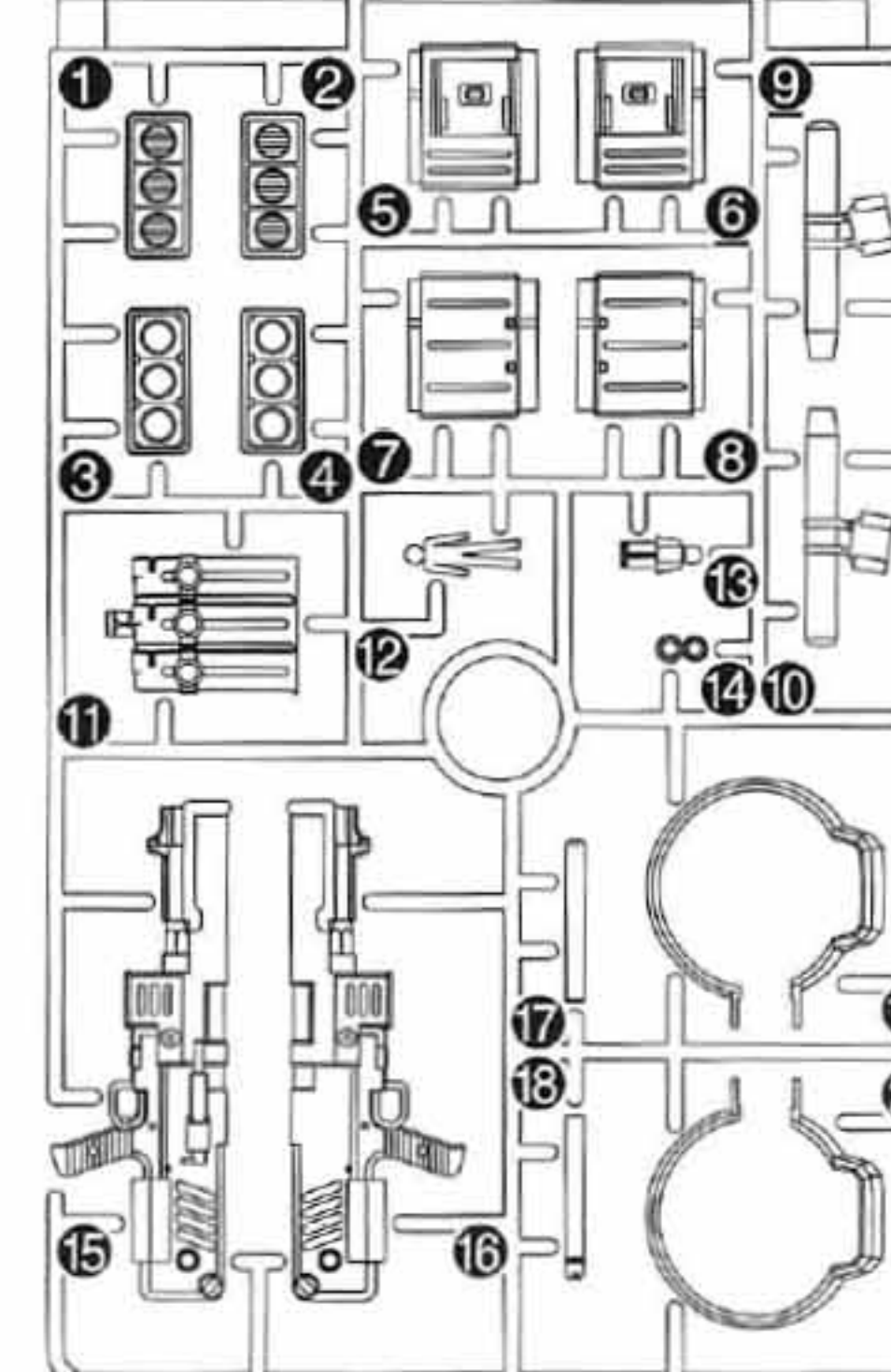
PC-125パーツ(グレー) (PE) PC-125 Parts (Gray)
