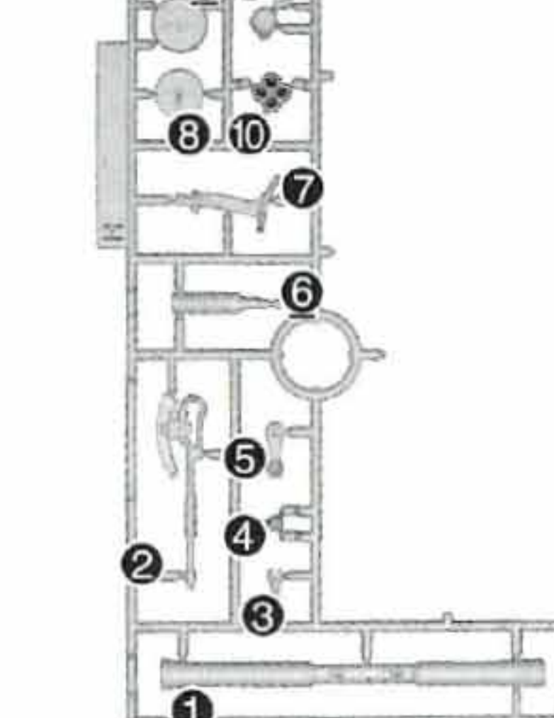
Hパーツ(ダークグレー) (PS)
