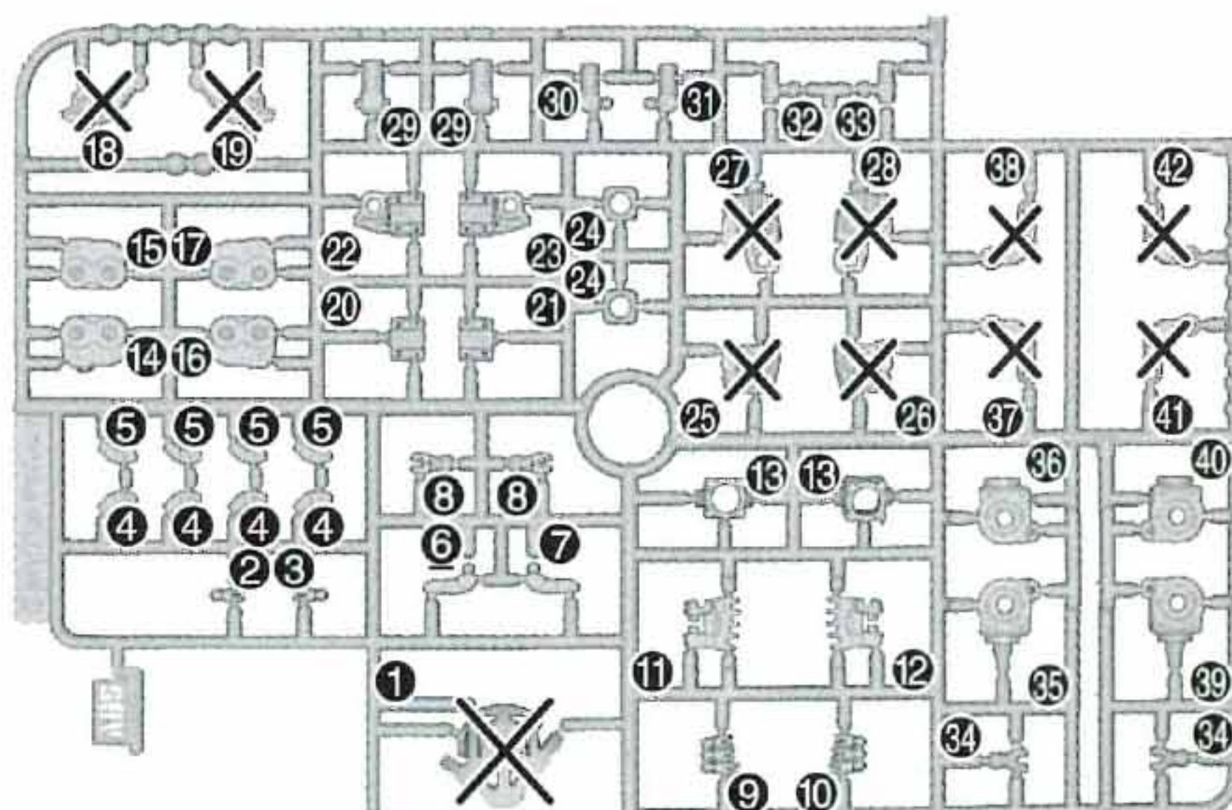
Gパーツ(ダークグレー) G Parts (Dark Gray) (ABS)
