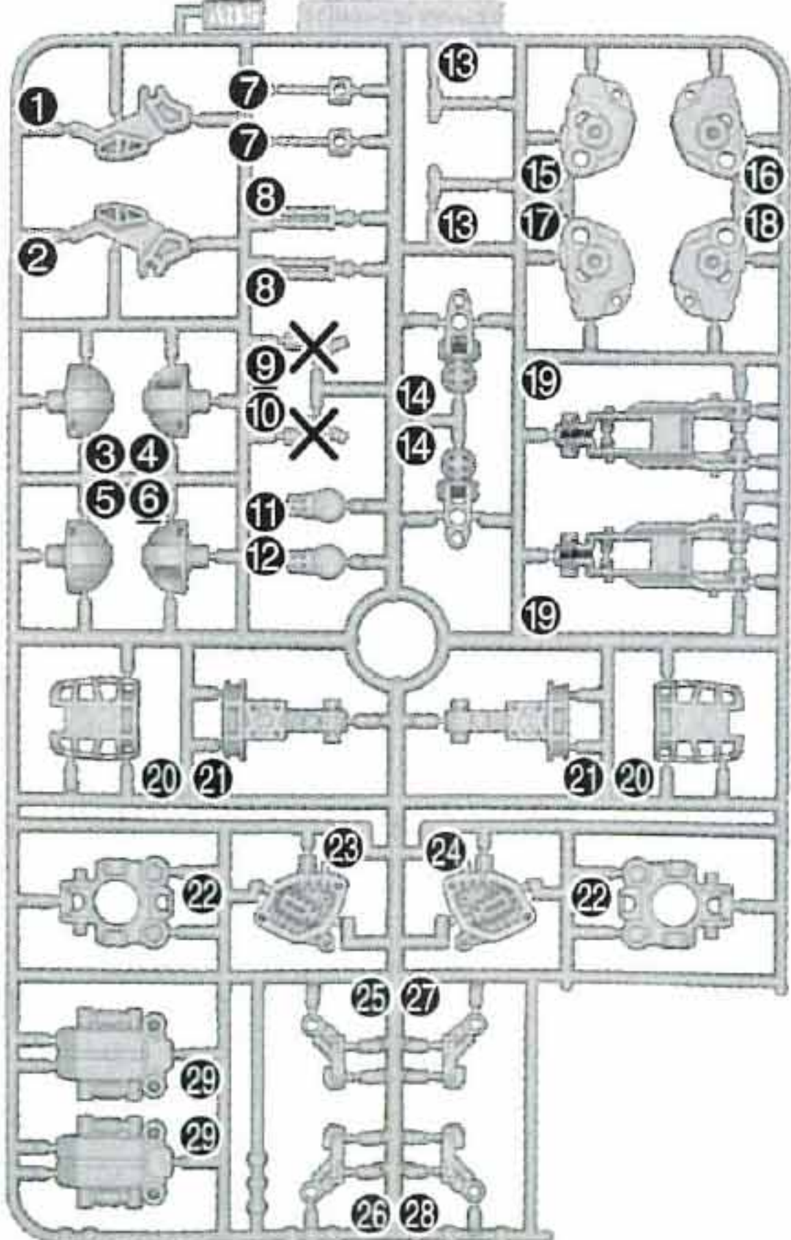
Hパーツ(ダークグレー) H Parts (Dark Gray) (ABS)
