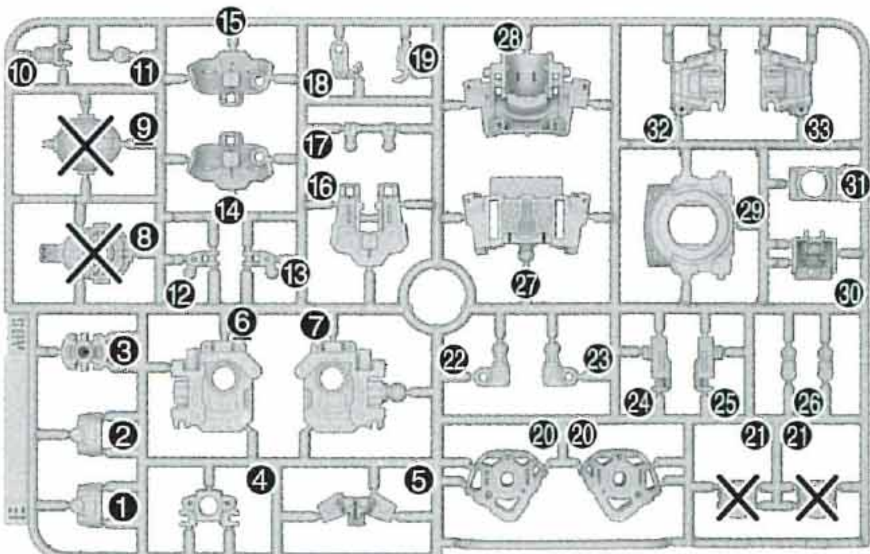
Eパーツ(ダークグレー) E Parts (Dark Gray) (ABS)
